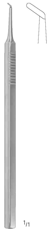
DEITZ 9,5 cm/3 3 / 4 " KP 548/50 0,50 mm KP 548/55 0,55 mm
